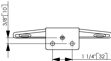
HOLE PATTERN GABARIT DE PERÇAGE
